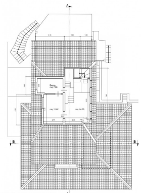
PIANTA PIANO SECONDO 1:100
