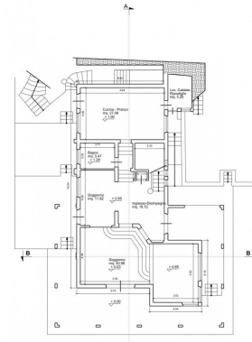
PIANTA PIANO TERRA 1:100
