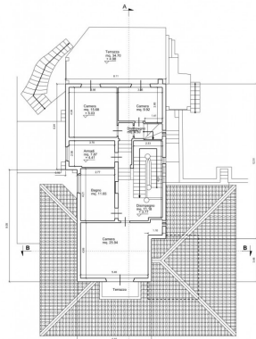
PIANTA PIANO PRIMO 1:100
